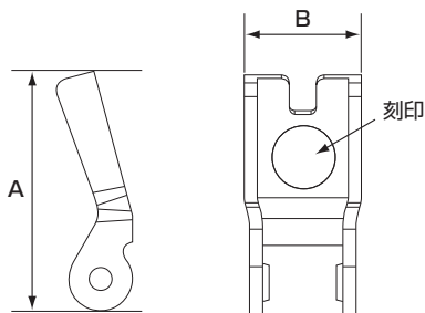
図22 外れ止め寸法
