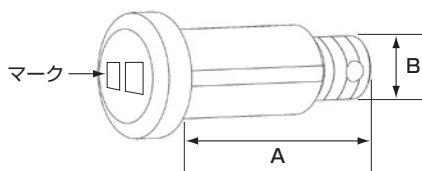
図23 チェーン止めボルト寸法
