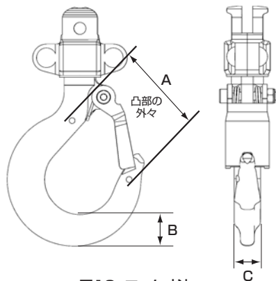
図13 フック寸法
