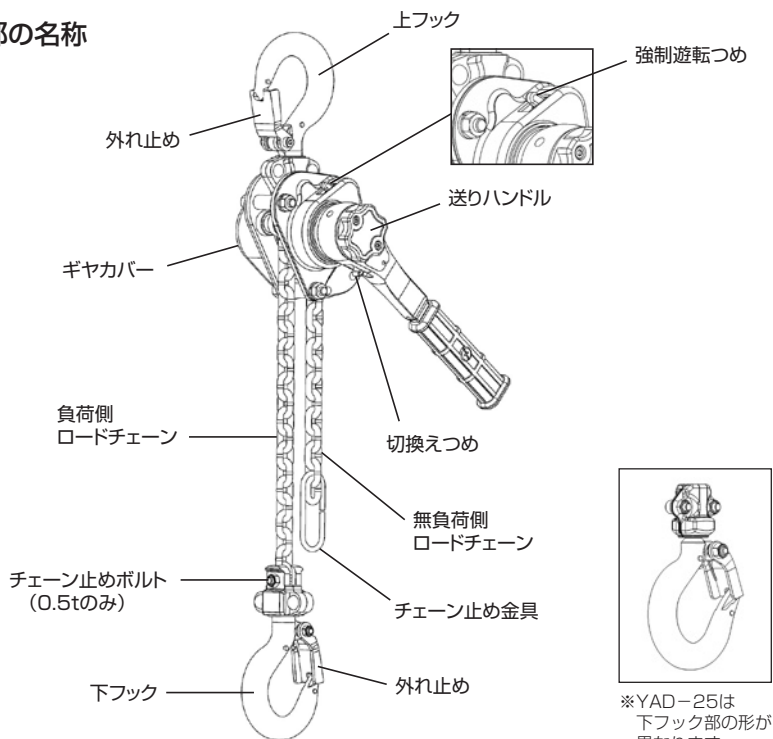
図1 各部の名称
