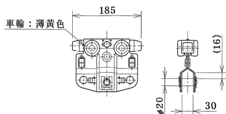
HB110S シングルトロリ (定格荷重 500kgまで)
