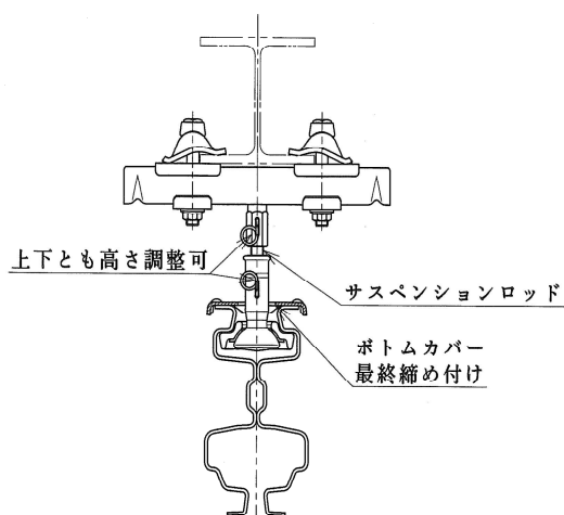
HB250 スタンダードサスペンション
