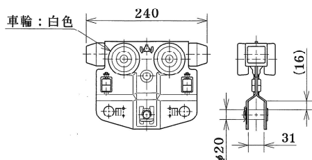
HB150S-250 シングルトロリ (定格荷重 630kgまで)
