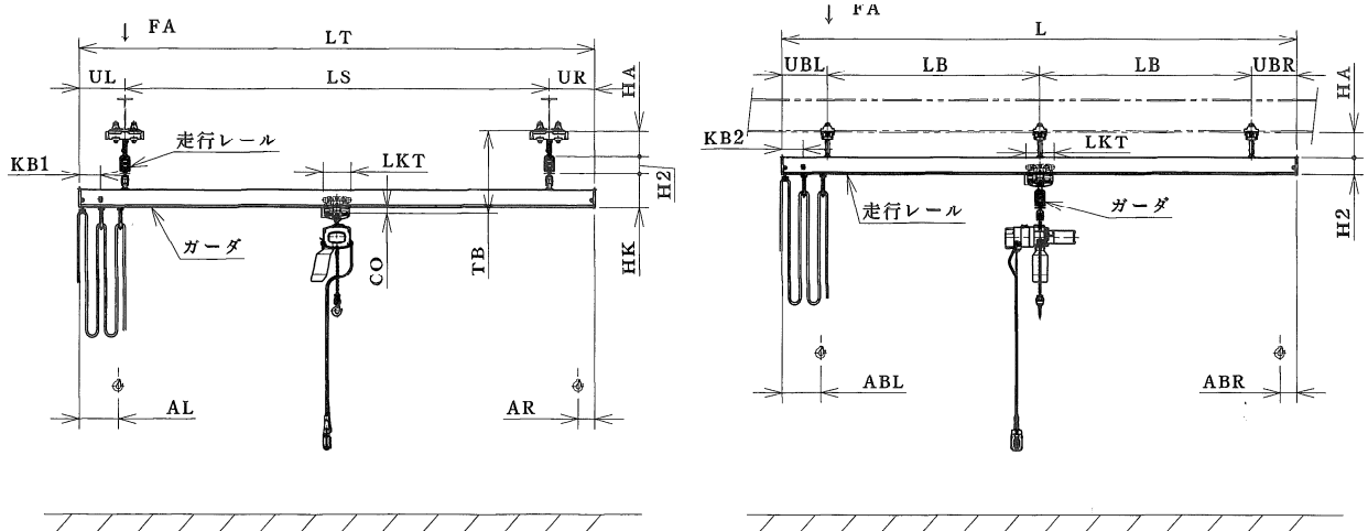
レール張り出し、トロリ巾 関係寸法表
