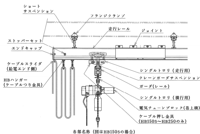
各部名称 (図はHB150Sの場合)
