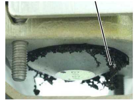
長い糸状のゴムがはみ出した状態
