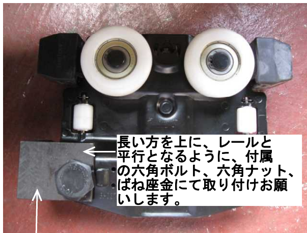
ケーブル押し金具
