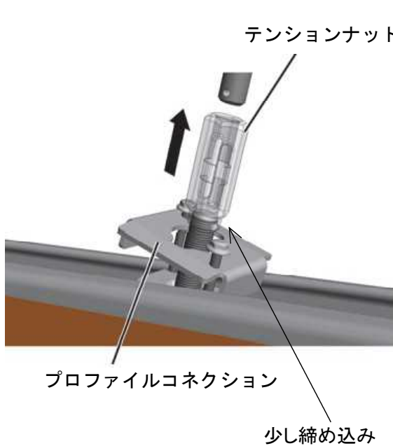
ショートサスペンション XS、S の場合
