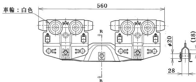
HB150S-250 ダブルトロリ (定格荷重 1tまで)
