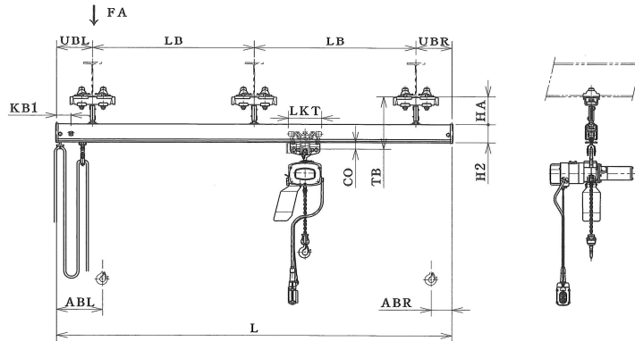
TB (天井取付底面～上フック掛け上面まで) 関係寸法表
