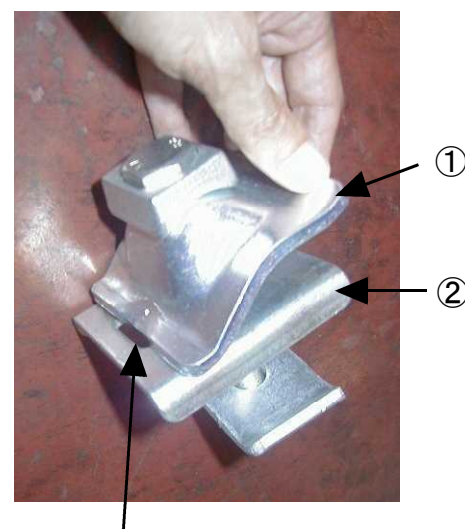
下ランププレートの穴へ引っ掛ける
