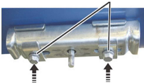
フランジランプのボルト 締め付けトルク150Nm
