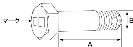
図15 チェーン止めボルト寸法
