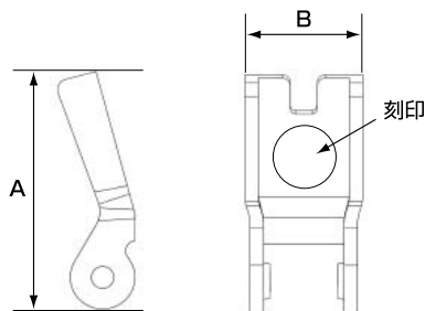
図14 外れ止め寸法
