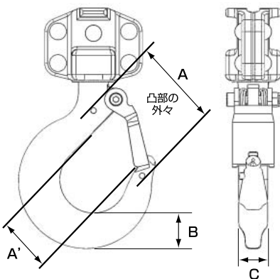
図13 フック寸法
