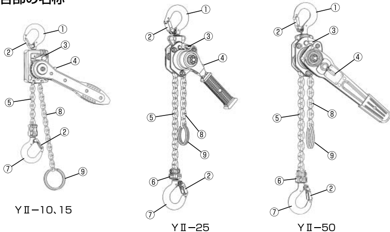
図1 各部の名称
