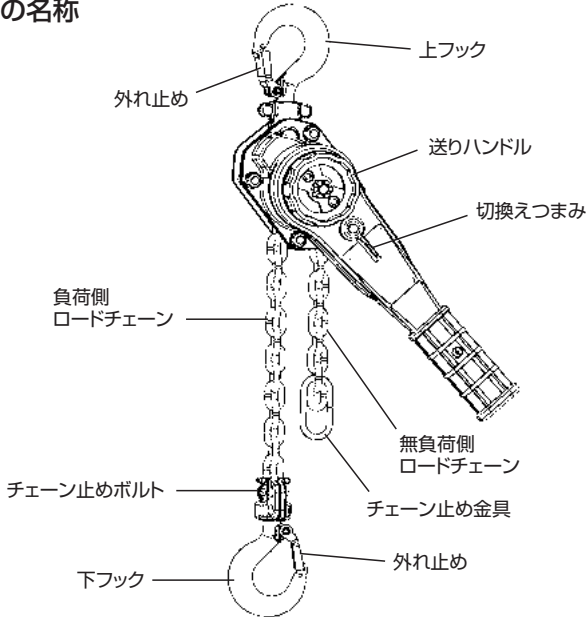
図1 各部の名称
