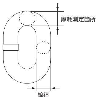
図18 線径
