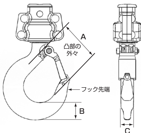
図14 フック寸法
